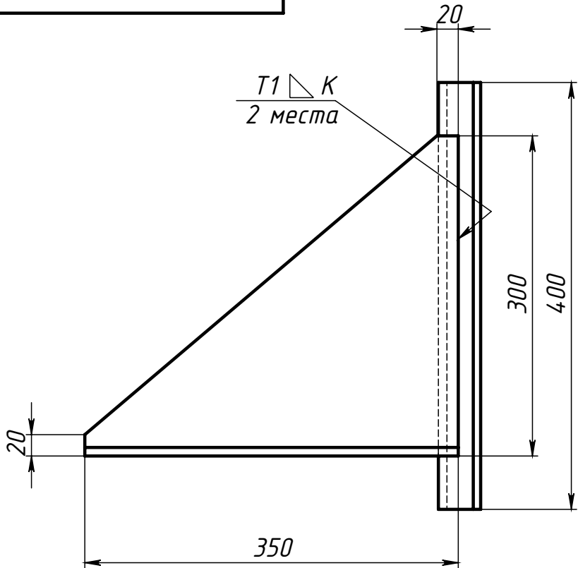
Поз.1 (Основание)
