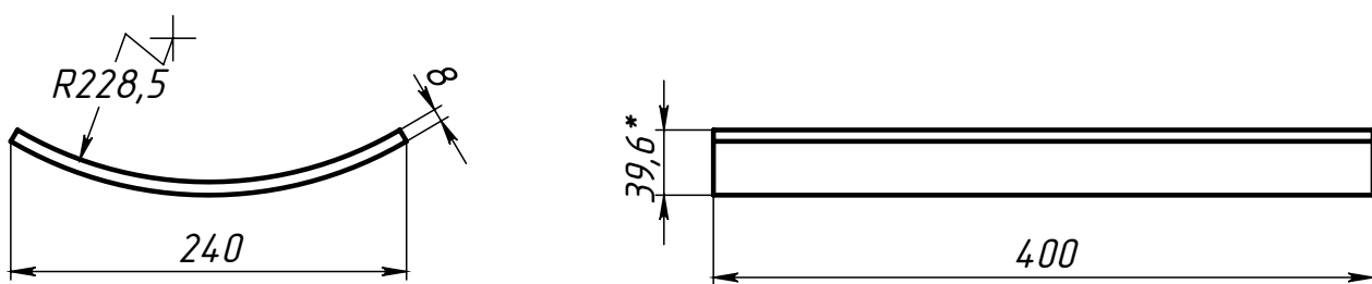
Поз.3 (Ложемент)
