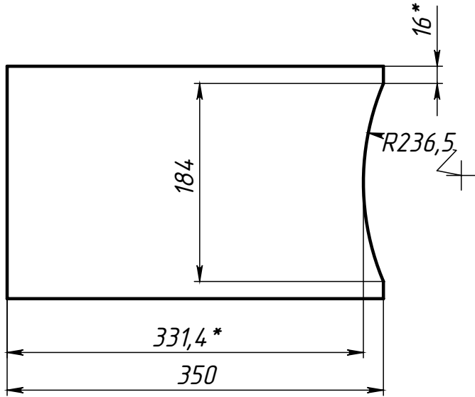
Поз.1 (Основание)
